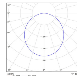
Krivka vyžarovania
